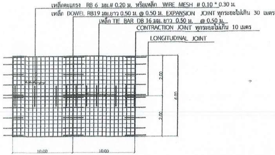
แบบแปลนถนคอนกรีตเสริมเหล็ก
