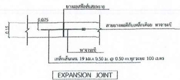
แบบแปลนถนคอนกรีตเสริมเหล็ก
