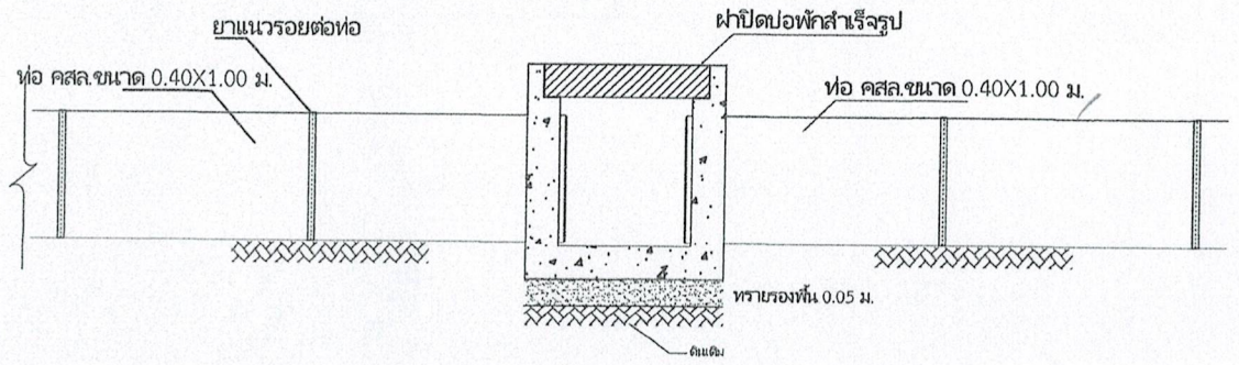
รูปตัดแนววางท่อพร้อมบ่อพักน้ำ
