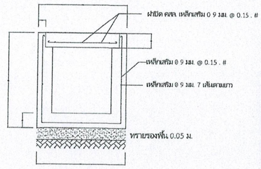
แปลนบ่อพัก
