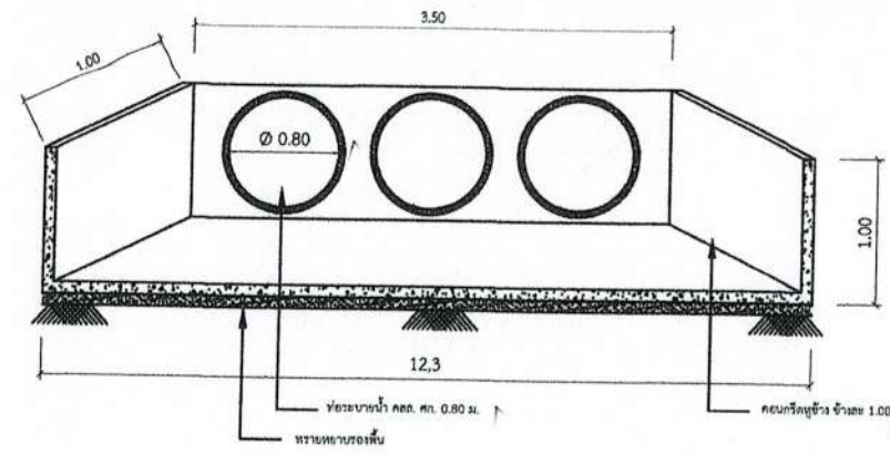
แบบแปลนแสดงการวางท่อ 3 แถว พร้อมหูช้าง
