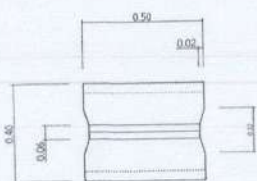
แปลนฝาร่องระบายน้ำ มาตราส่วน 0 : 0
