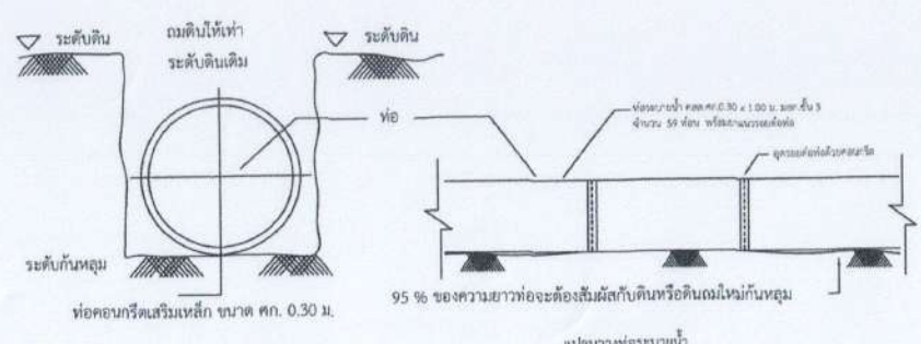
แปลนวางท่อระบายน้ำ
