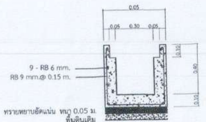
รูปตัดร่องระบายน้ำ มาตราส่วน 0 : 0
