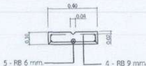
รูปตัดฝาร่องระบายน้ำ มาตราส่วน 0 : 0
