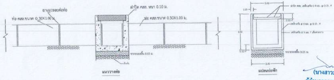
แปลนวางท่อระบายน้ำ
