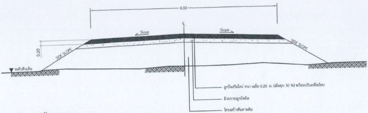
รูปตัดตามขวาง
