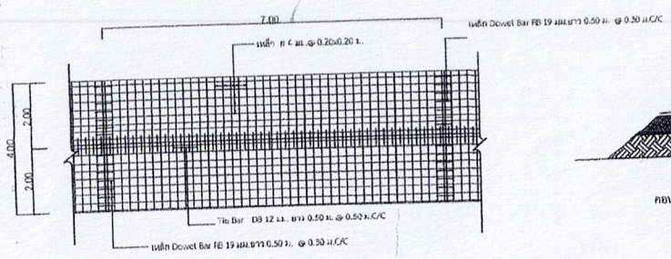
แปลนถนน คสล. แสดงการเสริมเหล็ก
