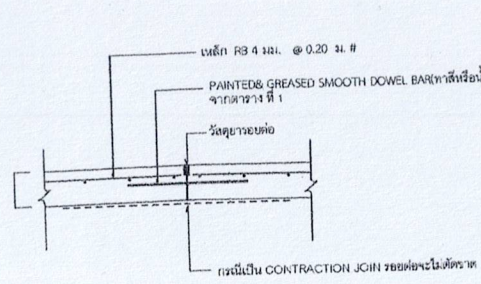
รูปตัดขยายรอยต่อ CONTRACTION JOINT
