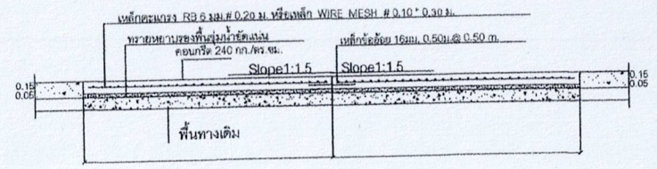
แปลนถนน คสล. รูปตัดตามขวาง
