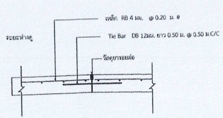
รูปตัดขยายรอยต่อ LONGITUDINAL JOINT
