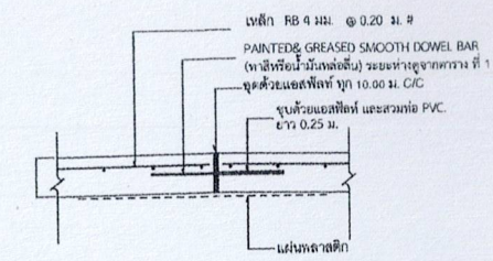
รูปตัดขยายรอยต่อ EXPANSION JOINT (ทุกระยะ 30 เมตร)
