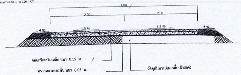
รูปตัด
